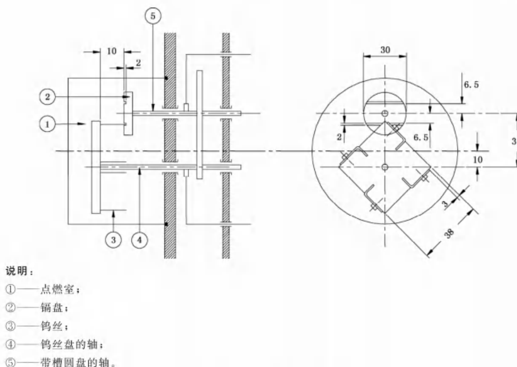
图 G.7 试验装置
