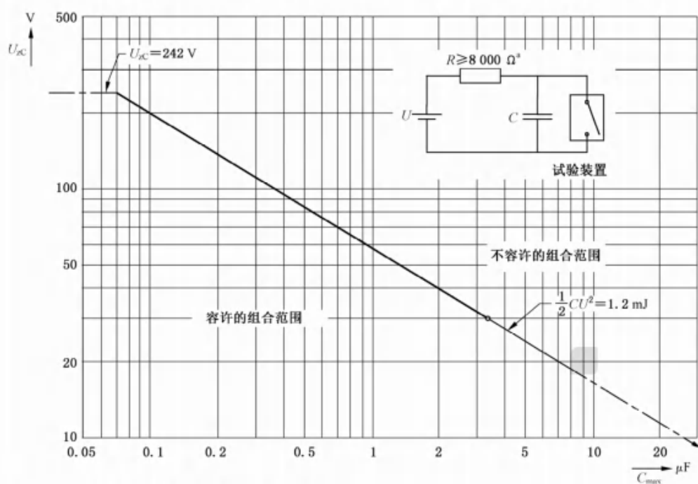
图 G.2 在乙醚蒸气和空气混合成的最易燃气体中电容电路上测得的 最大容许电压 U_{sc} 和电容 C_{max} 的函数关系
