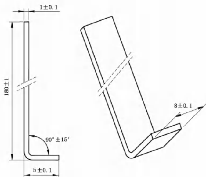
图7 试验钩(见 5.9.2.2)
