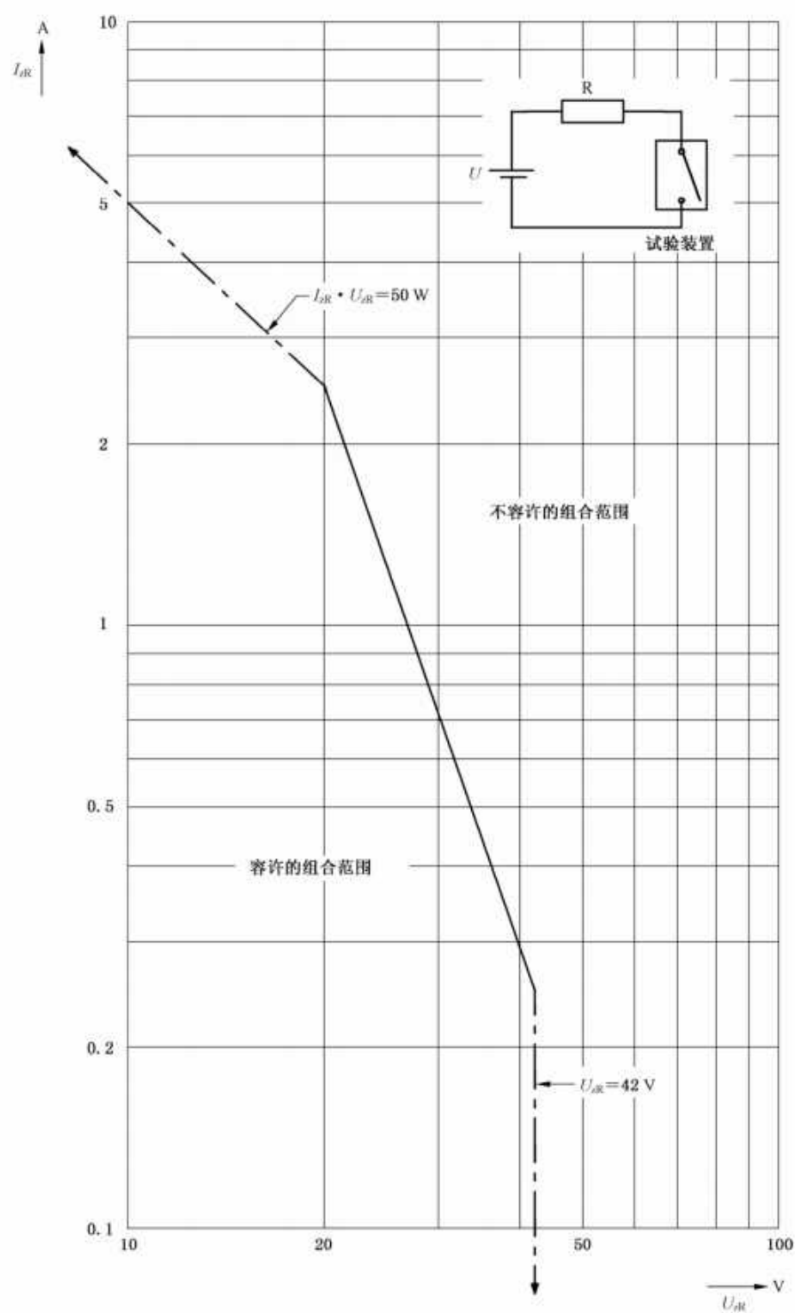
图 G.1 在乙醚蒸气和空气混合成的最易燃气体中纯电阻电路上测得的最大容许电流 I_{R} 和最大容许电压 U_{R} 的函数关系
