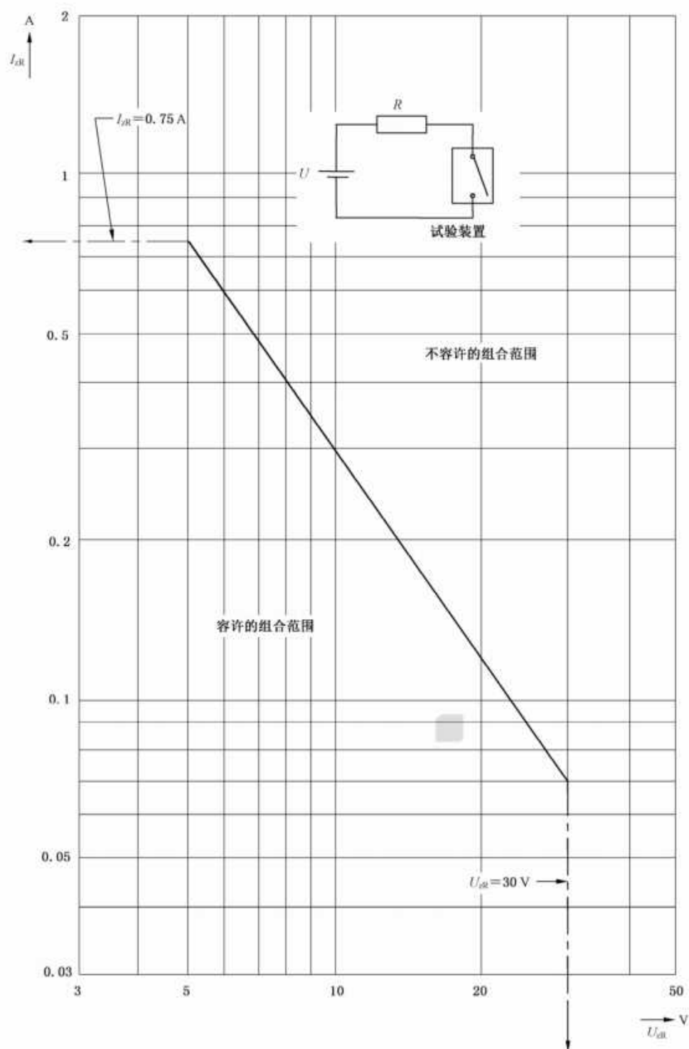
图 G.4 乙醚蒸气和氧混合成的最易燃气体中纯电阻电路上测得的最大容许电流 I_R 和最大容许电压 U_R 的函数关系
