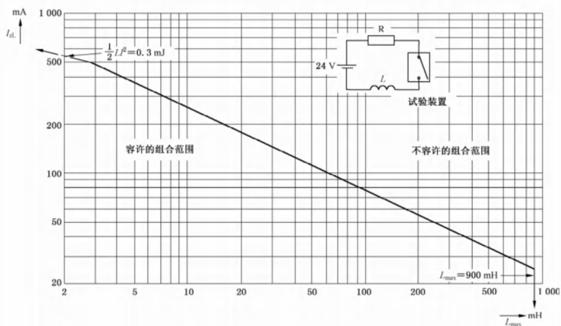
图 G.3 在乙醚蒸气和空气混合成的最易燃气体中电感电路上测得的 最大容许电流 I_{dL} 和电感 L_{max} 的函数关系
