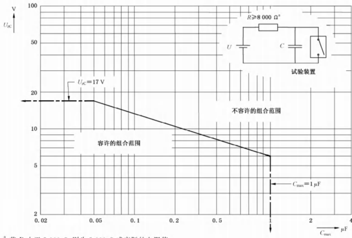
图 G.5 在乙醚蒸气和氧混合成的最易燃气体中电容电路上测得的 最大容许电压 U_{x\bar{C}} 和电容 C_{\max} 的函数关系
