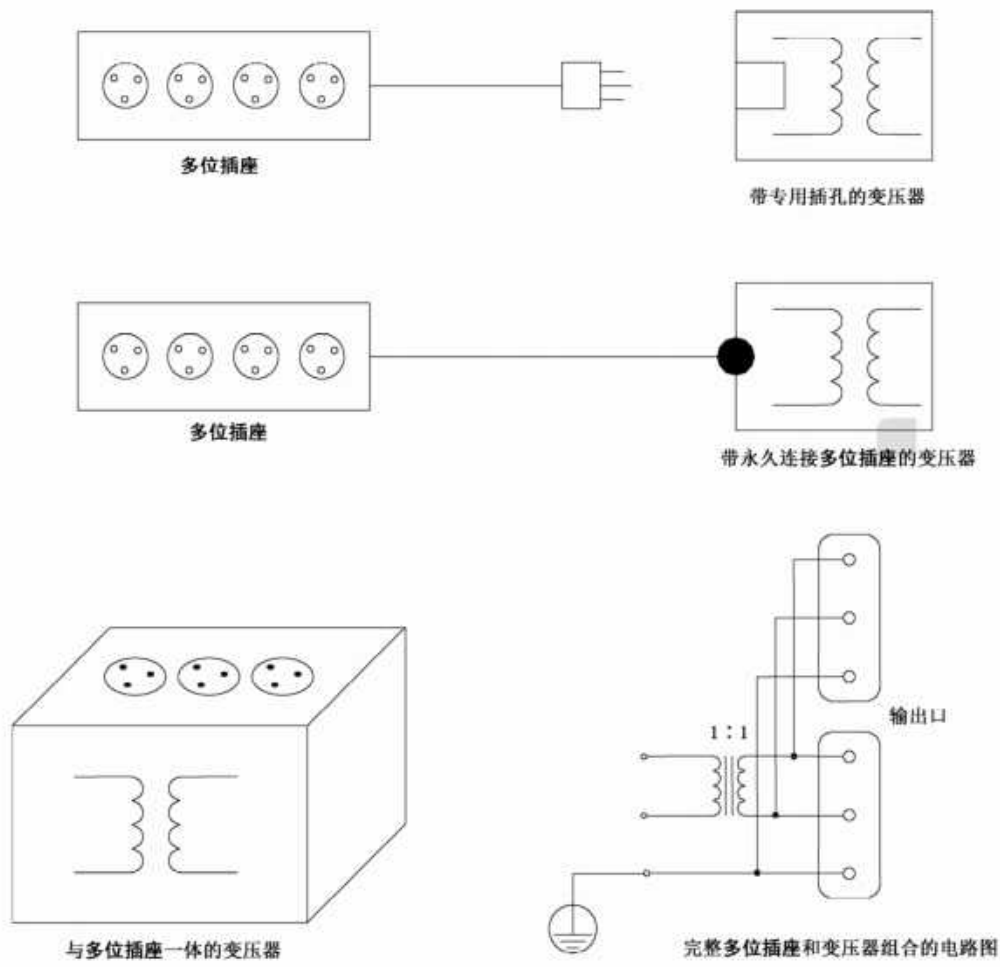
图 1.2 多位插座应用的实例
