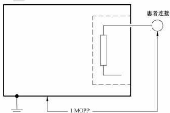
图 J.7 绝缘示例 7
