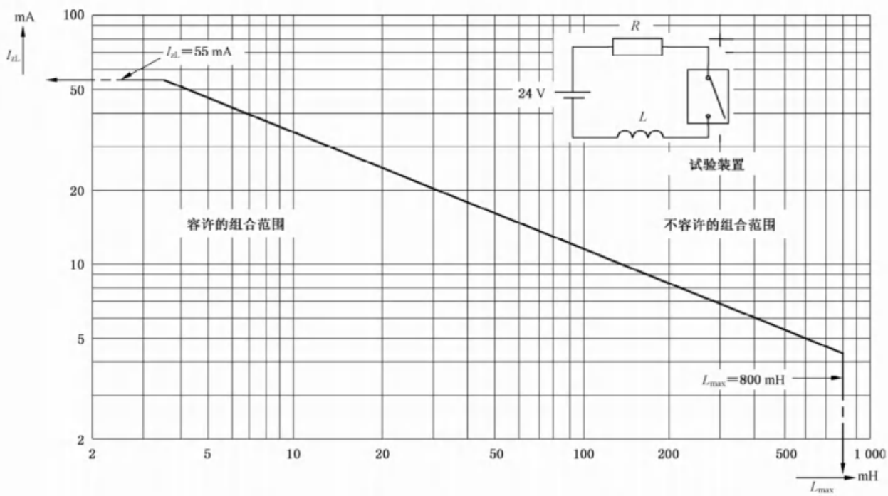
图 G.6 在乙醚蒸气和氧混合成的最易燃气体中电感电路上测得的 最大容许电流 I_{x\bar{L}} 和电感 L_{\max} 的函数关系
