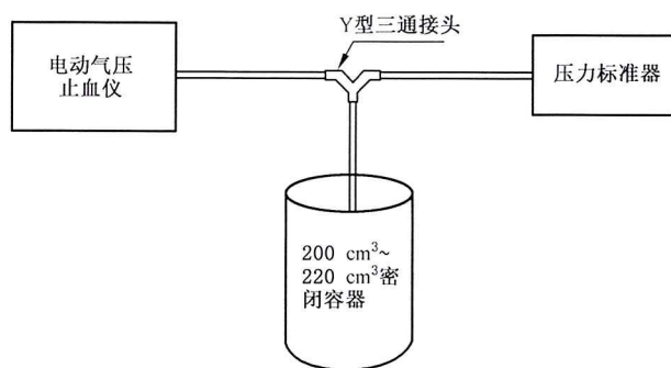
图 2 充气源测试示意图
