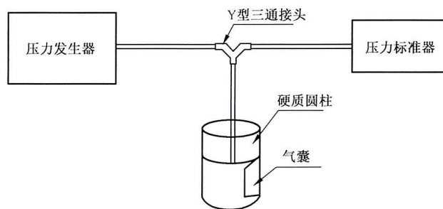
图 3 耐压力测试连接示意图
