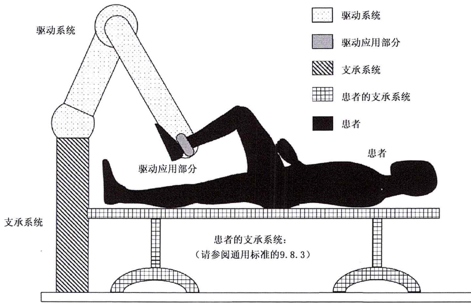
示例 1: 用于下肢的机械臂式 RACA 机器人
