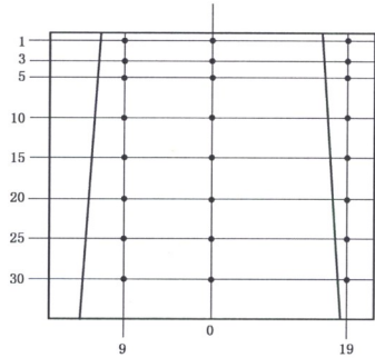
射野 25 cm×25 cm SSD=100 cm
