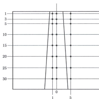
射野 5 cm×25 cm SSD=100 cm
