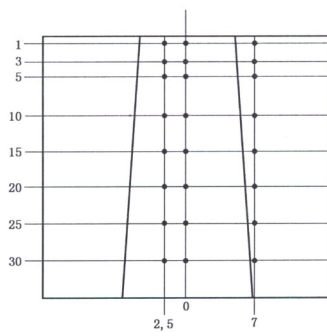
射野 10 cm×10 cm(在 SAD 位置) SSD=85 cm
