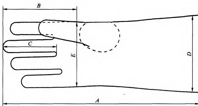
图 1 防护手套的内部尺寸
