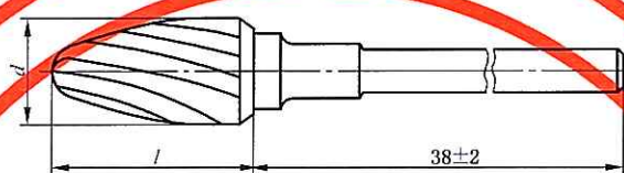
图 8 抛物面形
