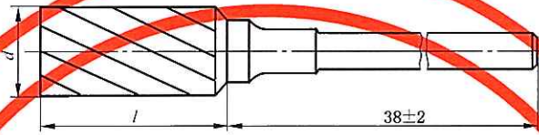
图 3 圆柱形
