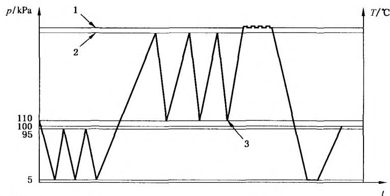
图 B.3 标准测试周期——高大气压排气
