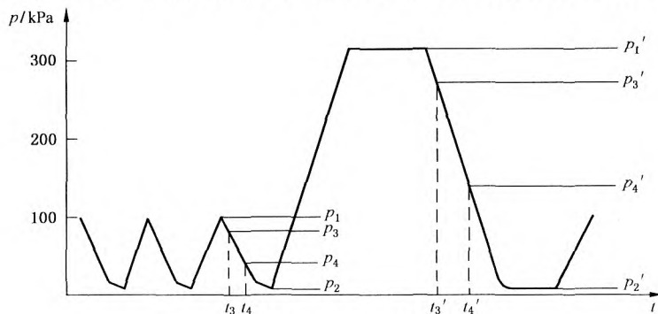
图 A.1 压力变化率的确定
