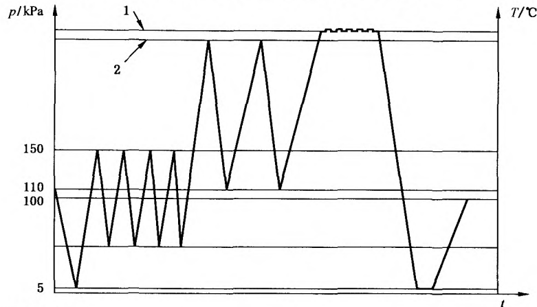
图 B.2 标准测试周期——跨大气压排气
