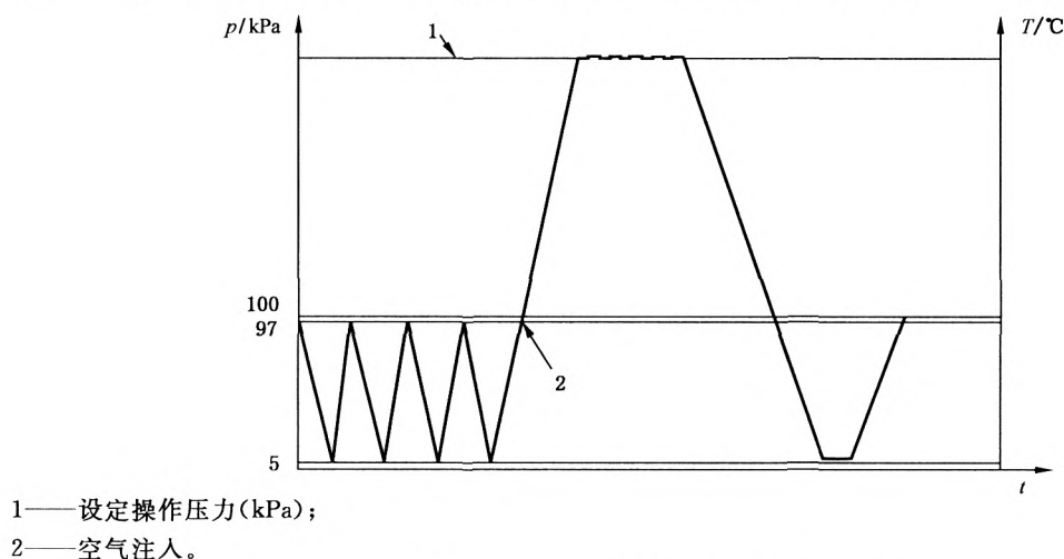
图 B.1 标准测试周期——低大气压排气
