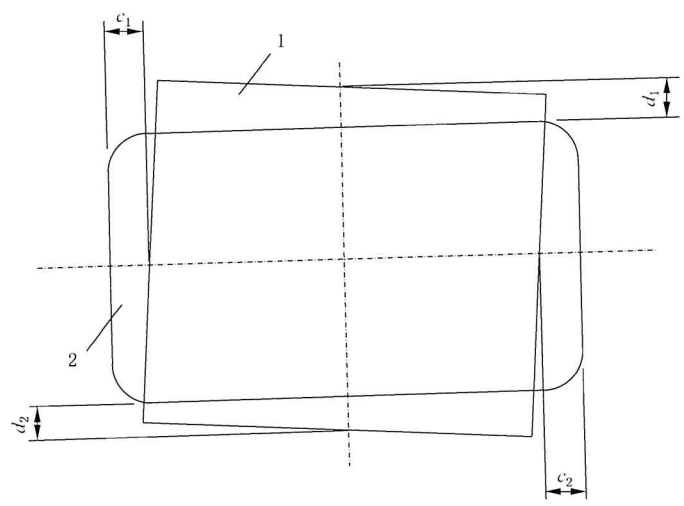
图 203.102 覆盖影像接收区域的偏差
