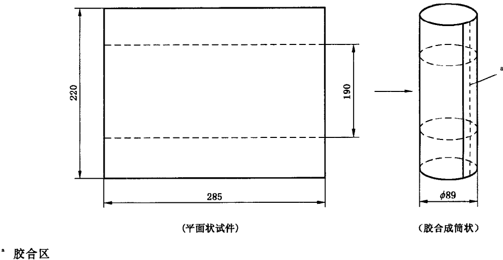
图 4 试件
