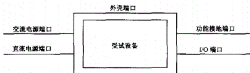
图 1 端口实例
