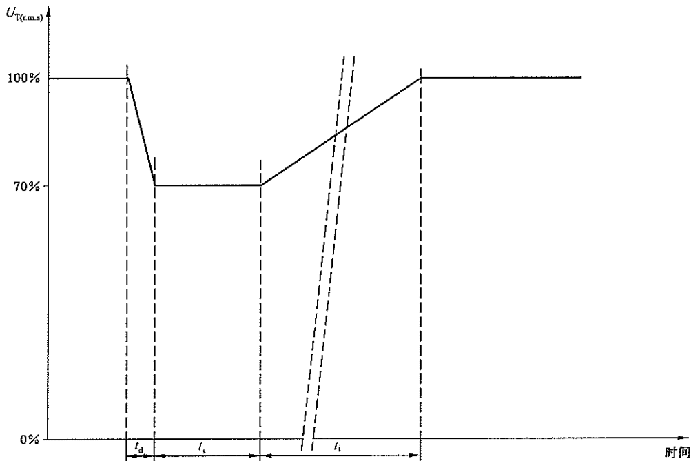
图 2 电压变化
