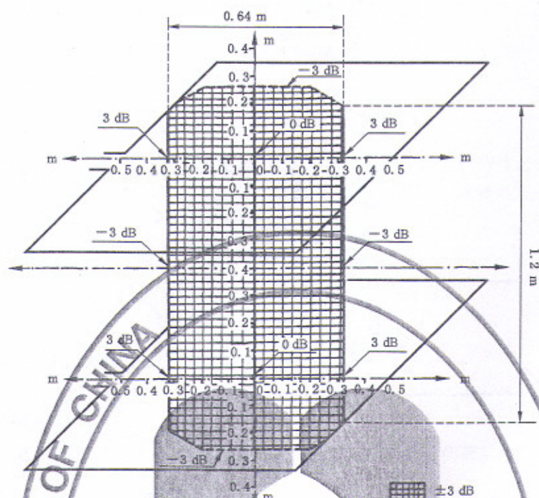
图 B.5 两个相距 0.8 m 的正方形(边长为 1 m)感应线圈在中央垂直平面上产生磁场的 3 dB 区域(垂直于线圈平面的分量)
