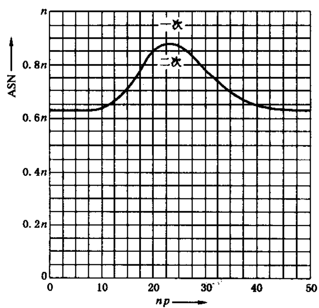
图 29 与判定数组[23,24]的设计值一次抽样方案 对应的的设计值二次抽样方案平均样本量曲线
