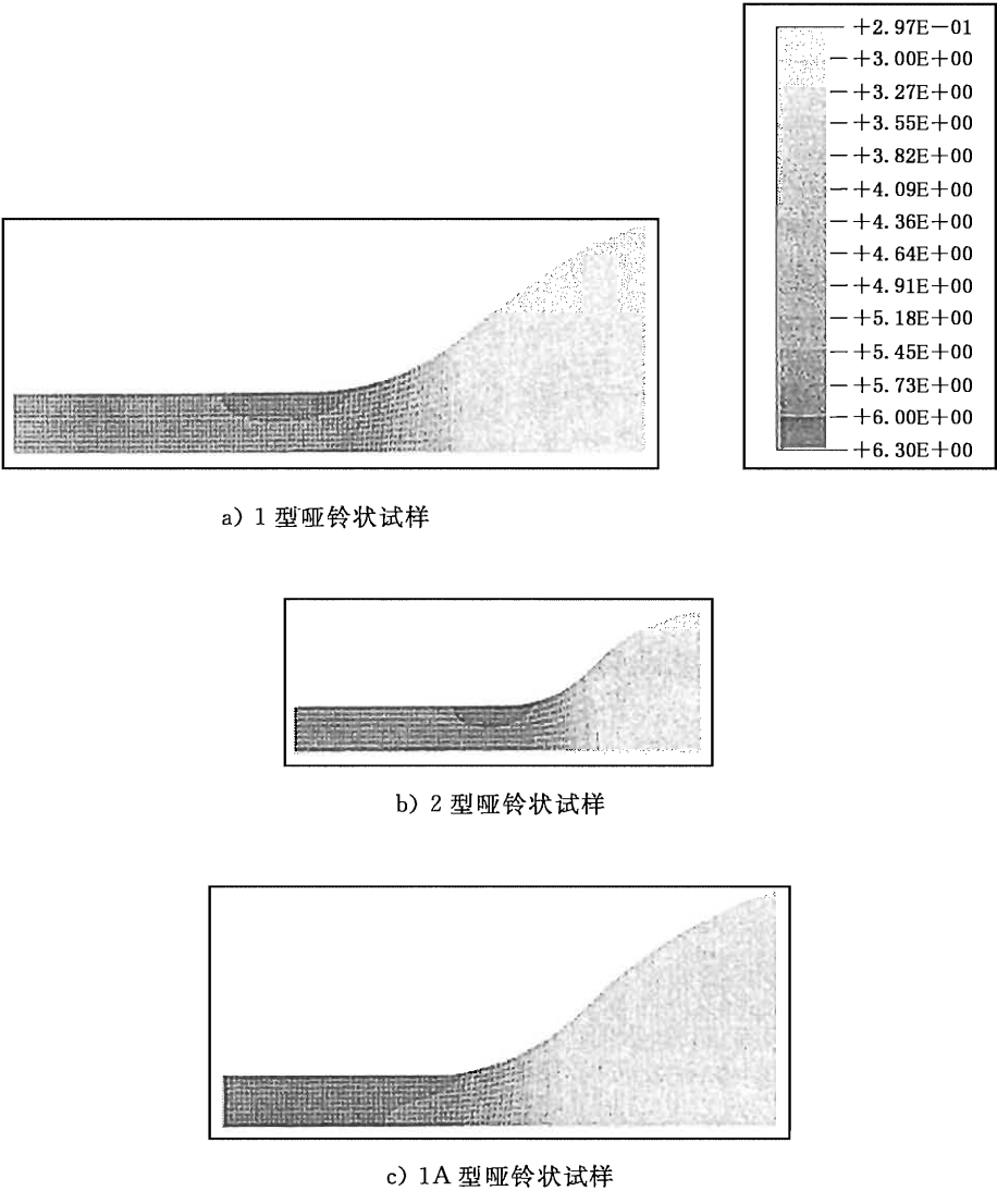
图 C.3 使用“ABAQUS”获得的应变分布实例
