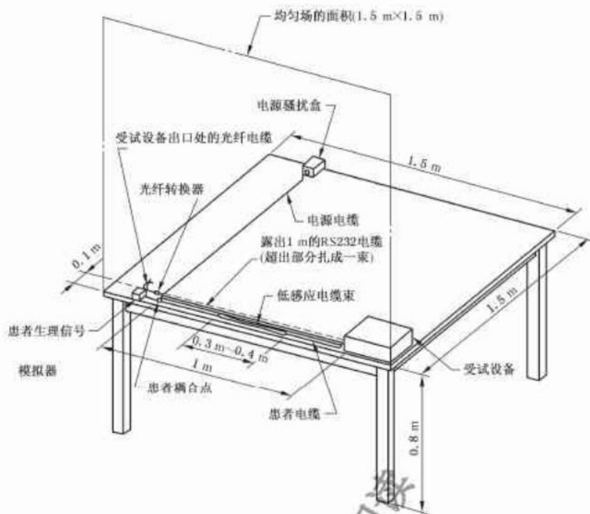
图 A.1 辐射抗扰度试验用电缆布置示例图
