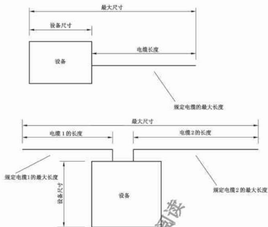
图 A.2 有一根电缆和两根电缆的设备最大尺寸示例图
