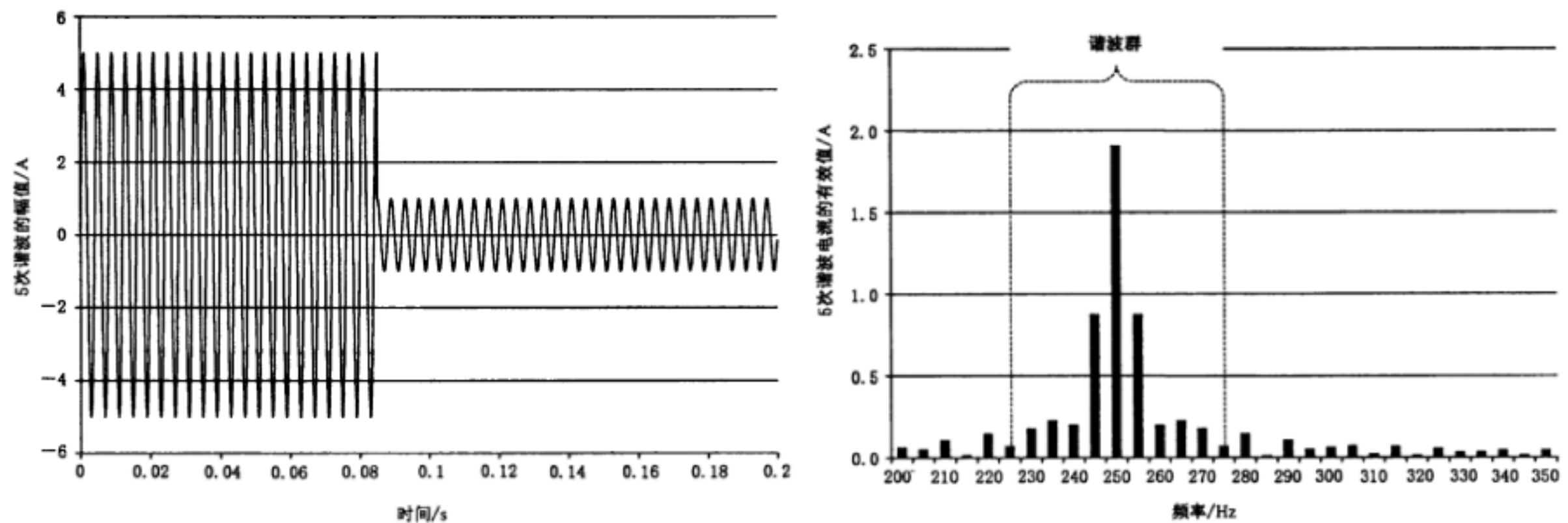
图 C.1 5 次谐波电流大波动
