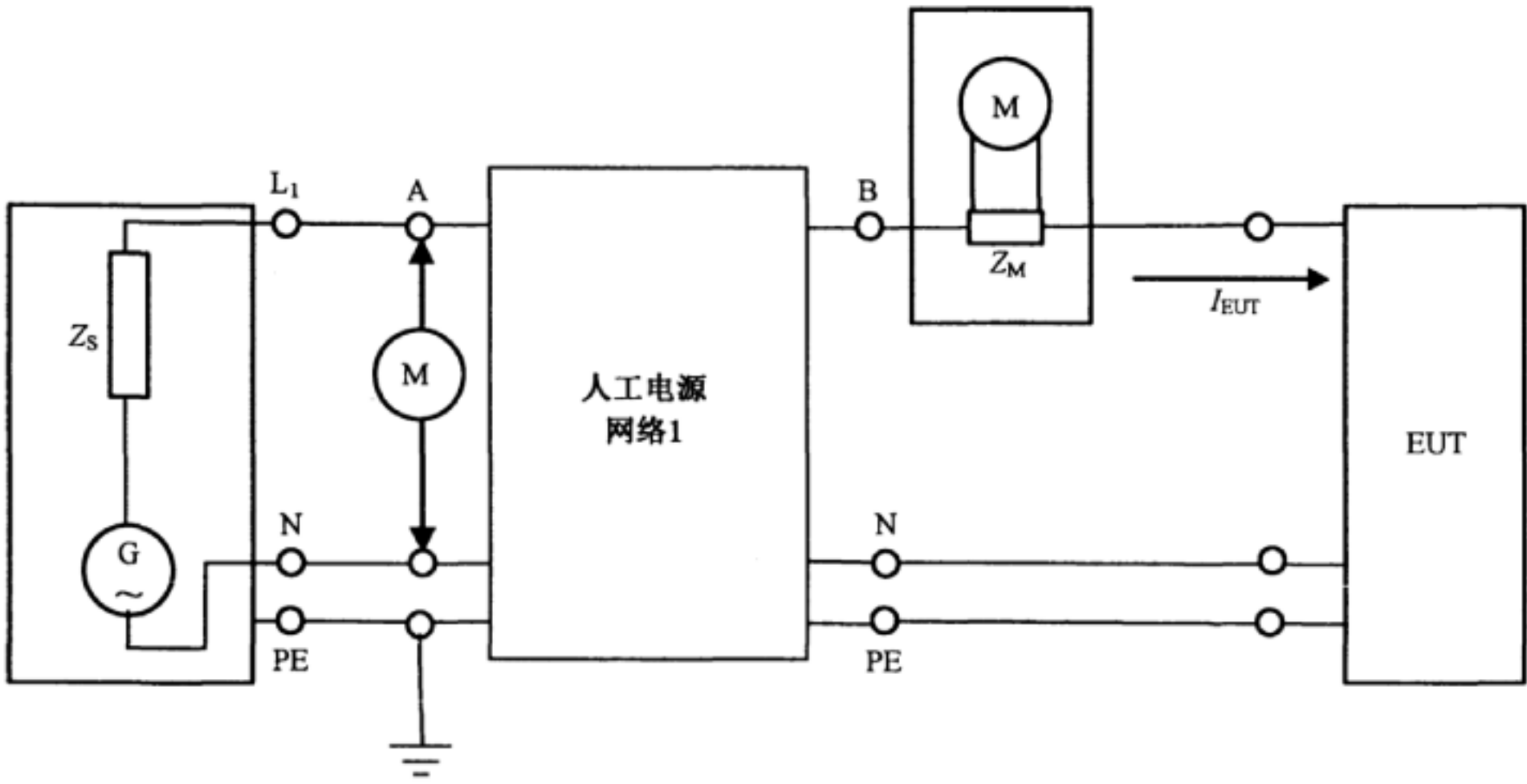
a) 单相测量布置
