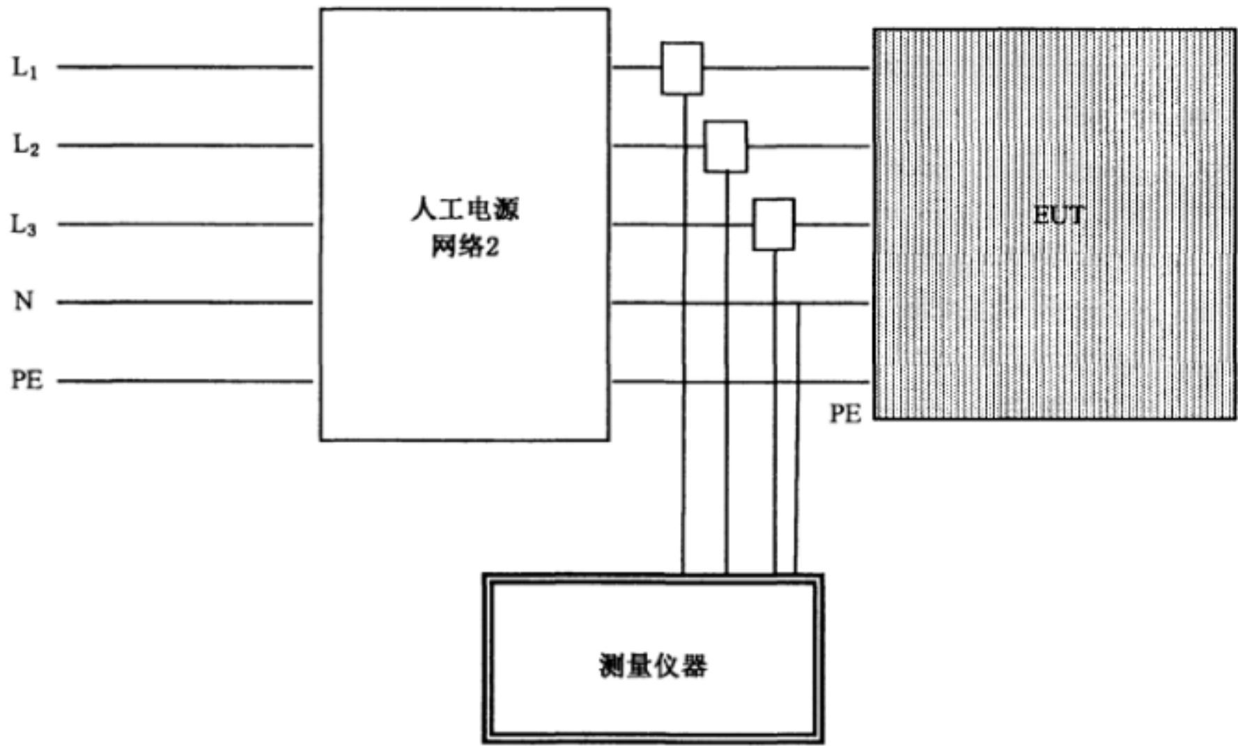
b) 三相测量布置
