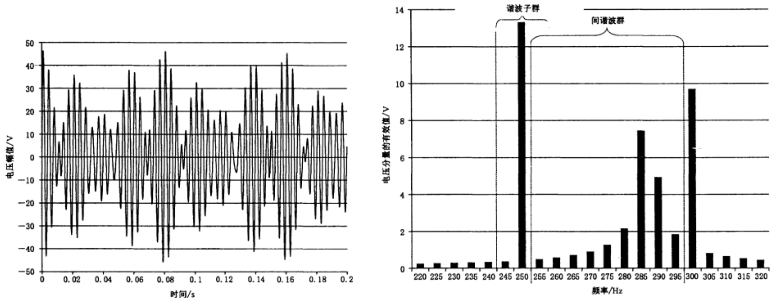
图 C.5 287 Hz 的间谐波以及 5 次和 6 次谐波
