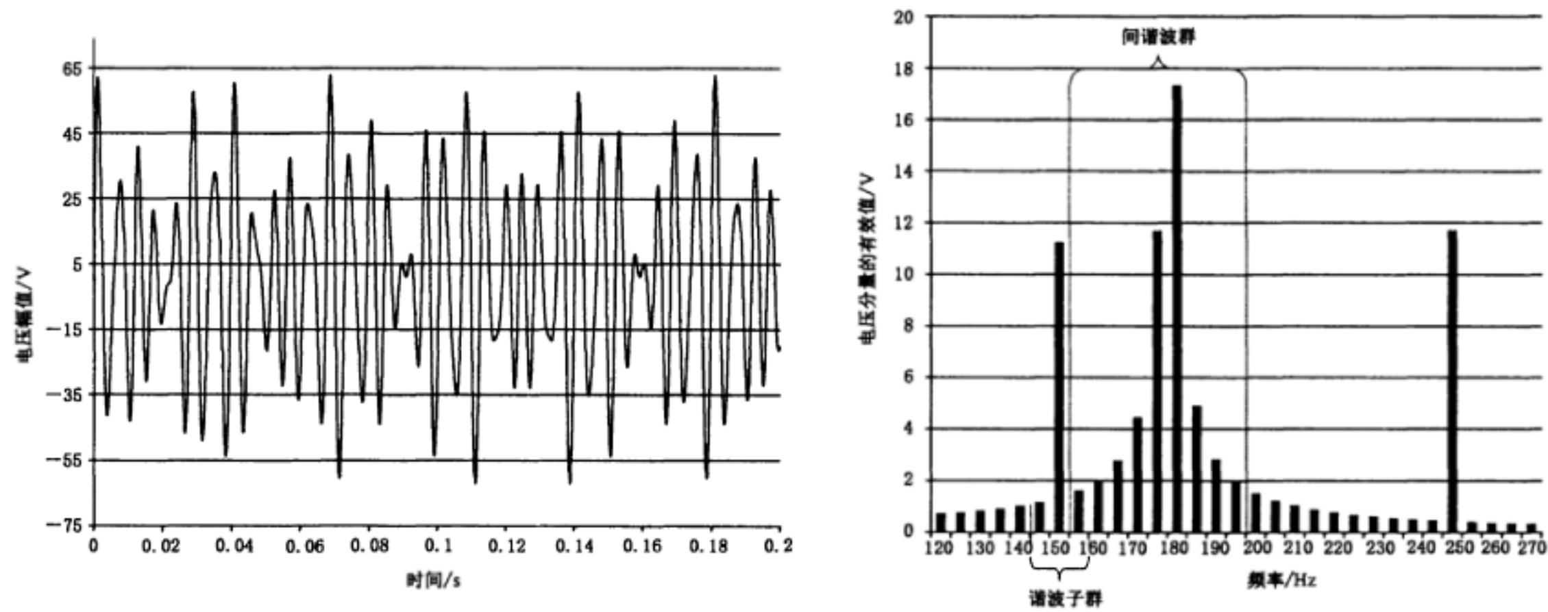
图 C.4 178 Hz 的通信信号以及 3 次、5 次谐波
