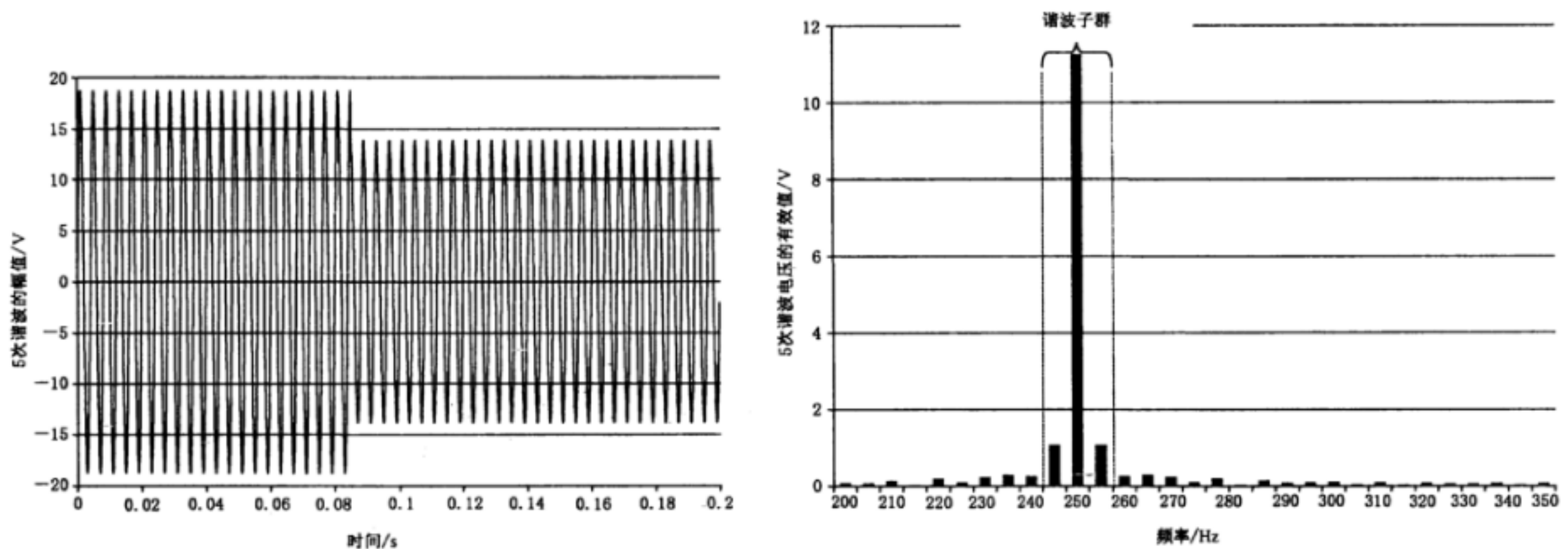
图 C.2 5 次谐波电压大波动
