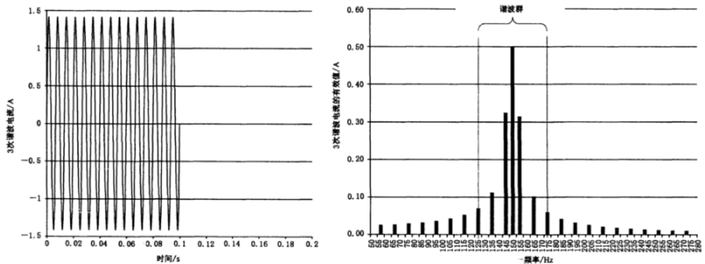
图 C.3 某微波器具波动的 3 次谐波电流
