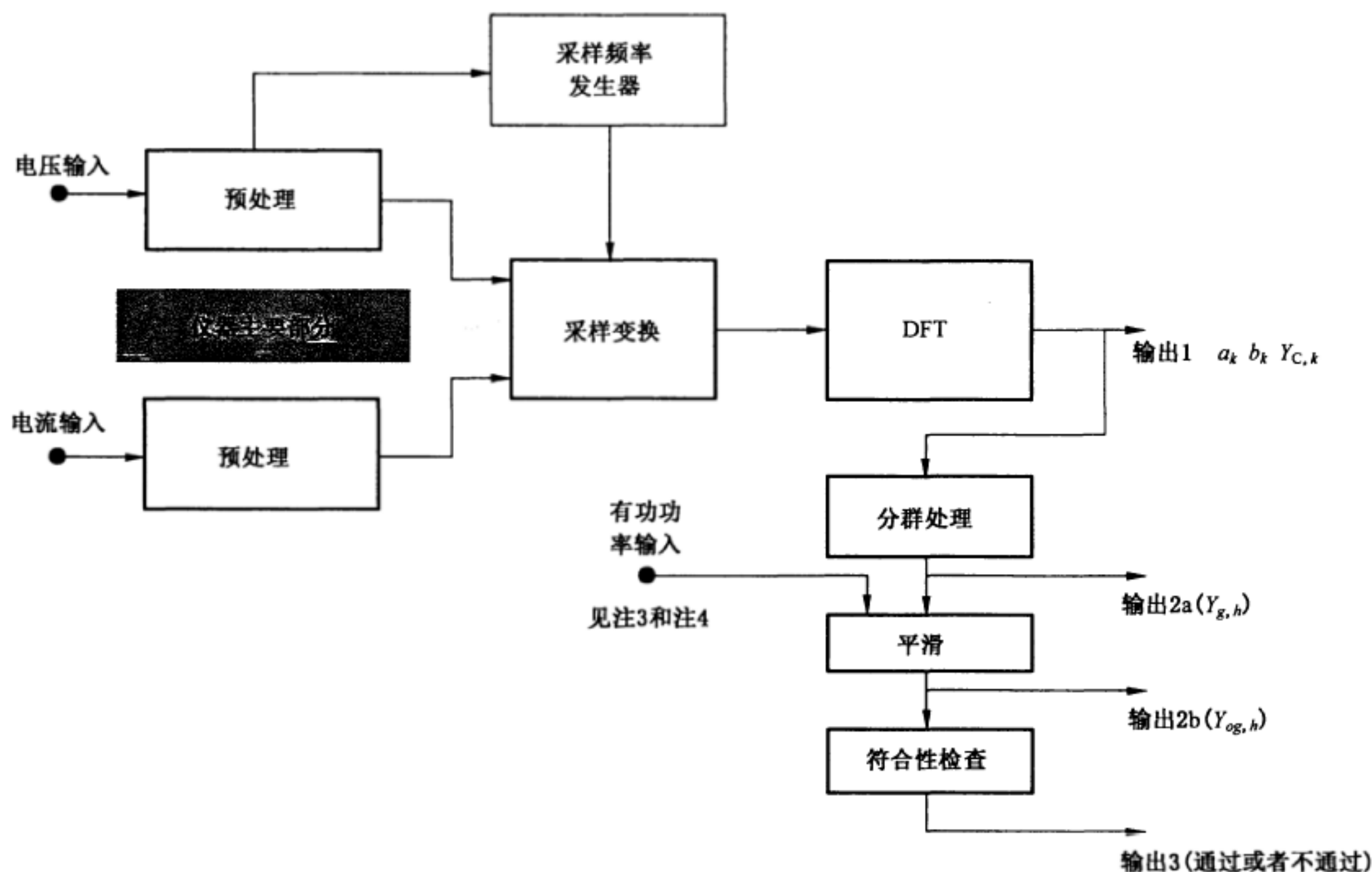
图 1 测量仪器的通用架构
