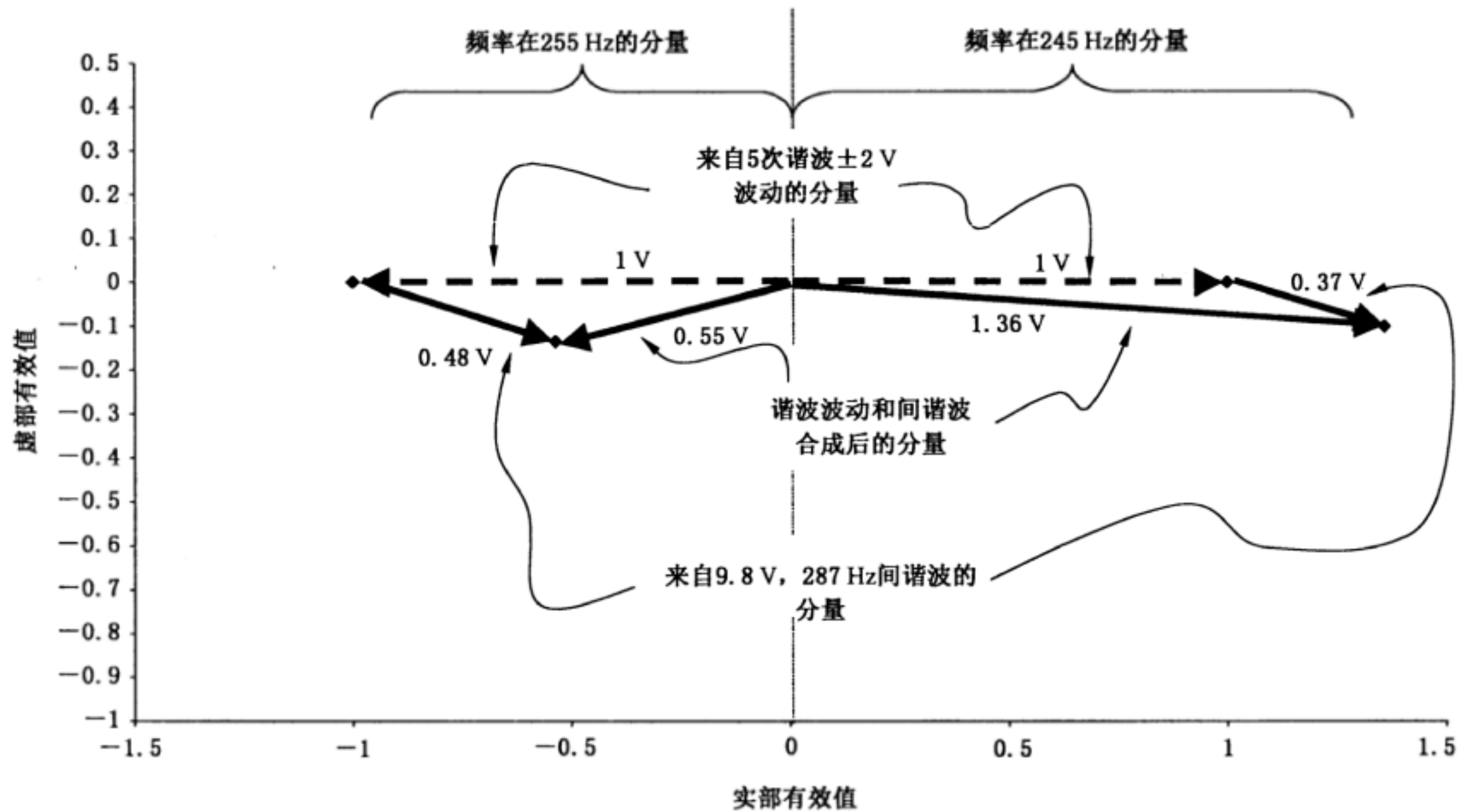
图 C.7 频率分别为 245 Hz 和 255 Hz 处的矢量
